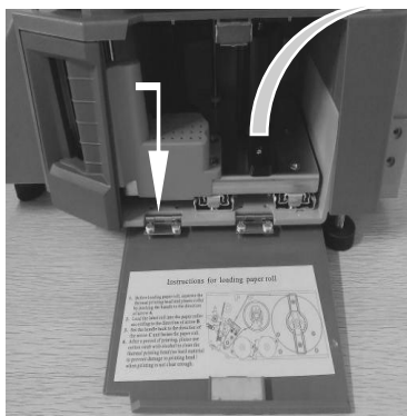
α. Ανοίξτε το πλαϊνό καπάκι και βγάλτε την κασέτα
